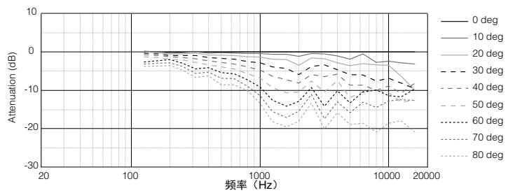
垂直离轴频率响应 (向上):
